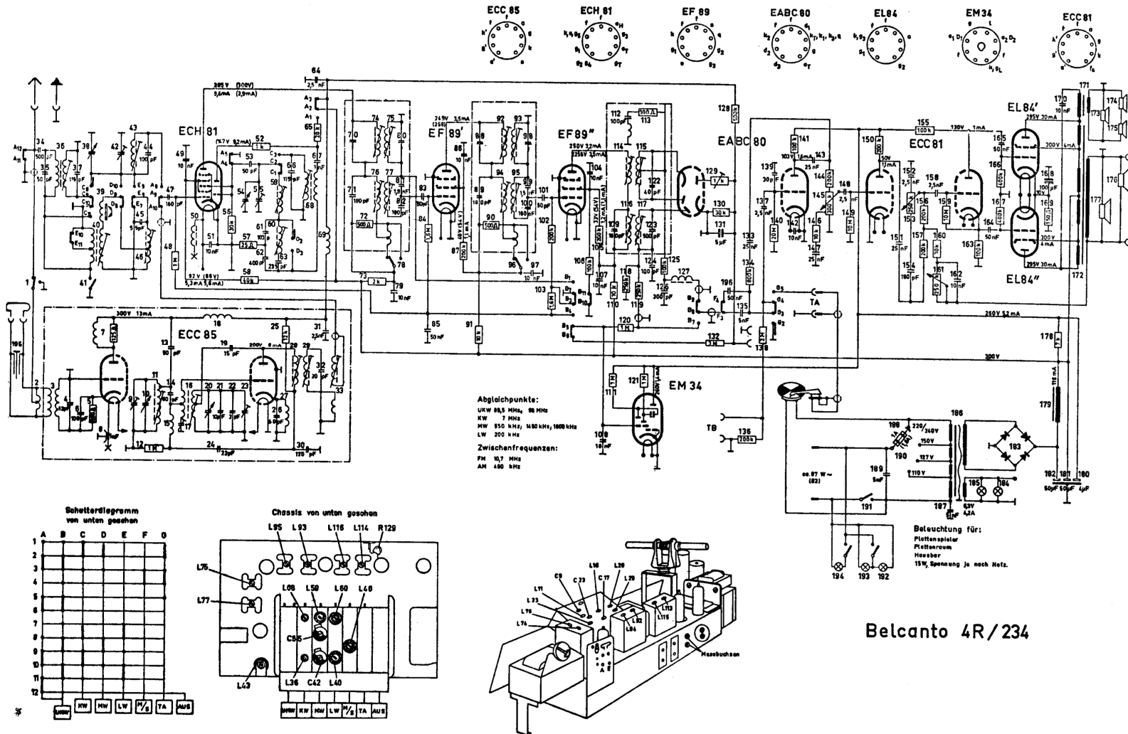
GRAETZ-SICART (Graetz Radio und Fernsehwerke, Altena) - Mod. Belcanto 4R/234. Apparecchio AM/FM ad alta fedeltà musicale, con sistema di riproduzione elettroacustica sistema 4R, con cinque altoparlanti a effetto stereofonico. Gamme d'onda: lunghe, medie e corte in AM e ultracorte in FM, MF/AM a 472 kc/s e MF/FM a 10,7 Mc/s. Potenza d'uscita indistorta 6 watt. Consumo 87 watt. (produzione 1956).
